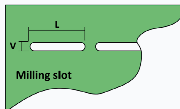
7915.591 TRACTOR-MILL2 depanellizzatore con pedale
